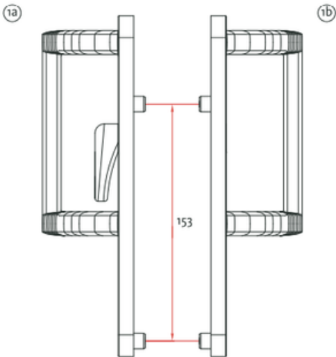
Manijón interior con leva
