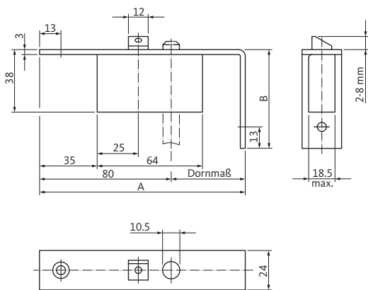
Schaltschloss B 1595 Stulpform: eckig/abgewinkelt
