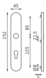
Round knob K1.1
