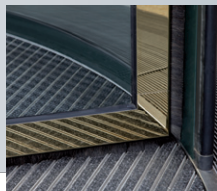
KONTORHAUS GEBR. HEINEMANN KG | HAMBURG | Typ GGG in Sonderausführung | vollautomatisch | Türflügel beplankt mit titanisiertem Edelstahl | spiegelpoliert | Decke aus einer Blechkonstruktion | ø 2860 mm
