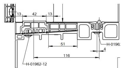
Festfeldverglasung
