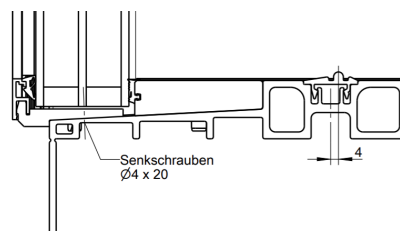
Schwellenverglasung
