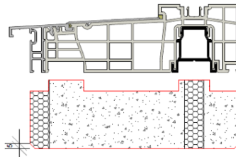
Kernverbundmaterial (KVM)
