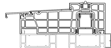
PVC
