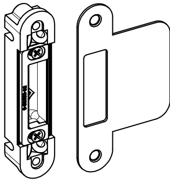
Zelfvergrendelende schoot Secury Automatic Secury 19xx/21xx Serie 21xx en Se-5321
