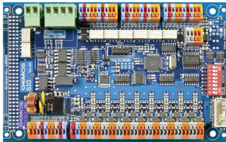
GEMOS I/O module zum Einbau in die GEMOS Box oder zur Montage auf der GEMOS Hutschienenträgerplatte
